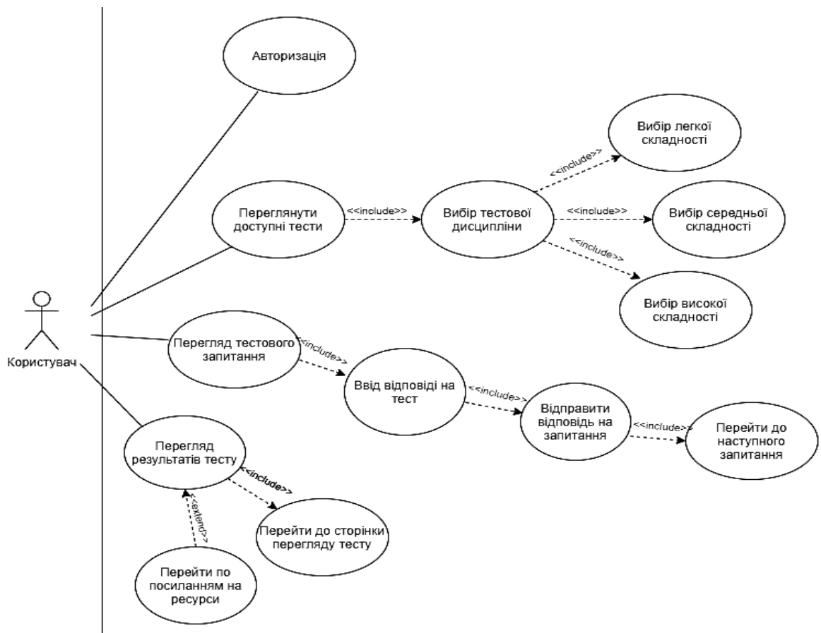
Рисунок 2. Діаграма функціональних можливостей системи
