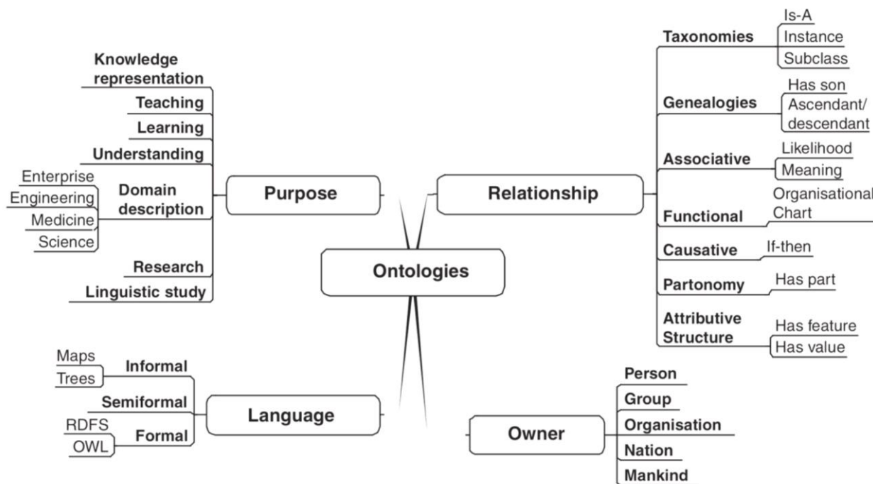
Рисунок 5. Приклад інтелект-карти 741
