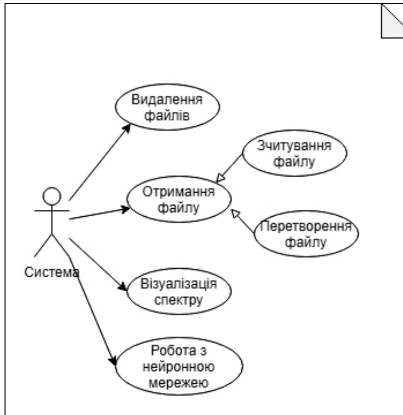
Рисунок 1. Діаграма прецедентів
